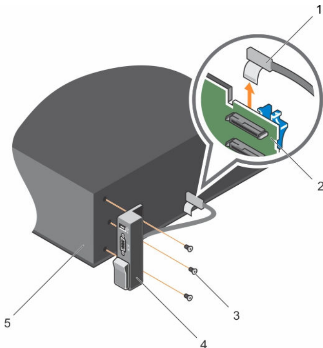
Abbildung 59. Entfernen und Installieren der E/A-Platine
