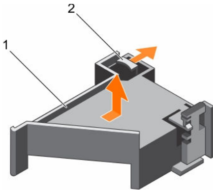
Abbildung 27. Entfernen und Einsetzen des PCIe-Kartenhalters
