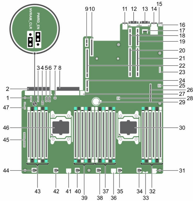
Abbildung 61. Jumper und Anschlüsse auf der Systemplatine
