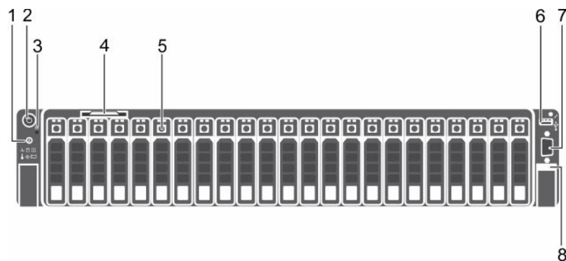
Abbildung 1. 2,5-Zoll-Festplatte oder SSD-Gehäuse
