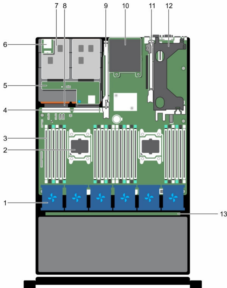
Abbildung 12. Das Innere des Systems – Dell XC730xd
