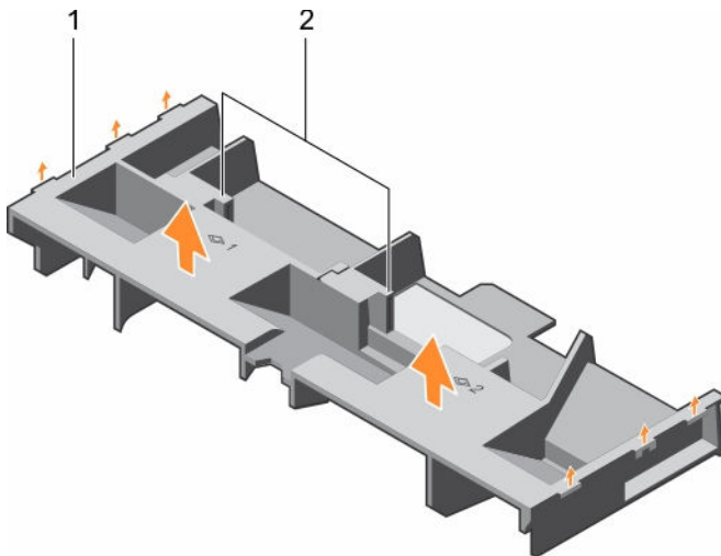
Abbildung 13. Entfernen und Einsetzen des Kühlgehäuses
