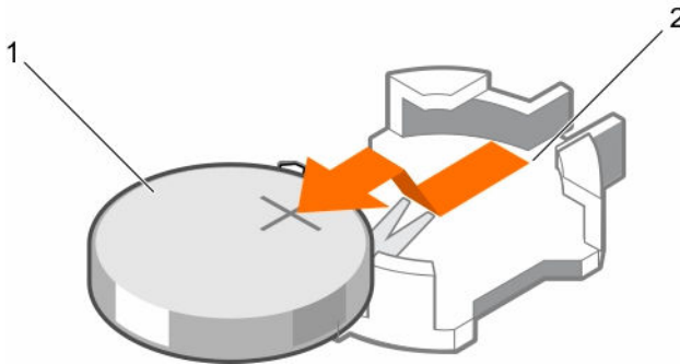
Abbildung 42. Entfernen der Systembatterie
