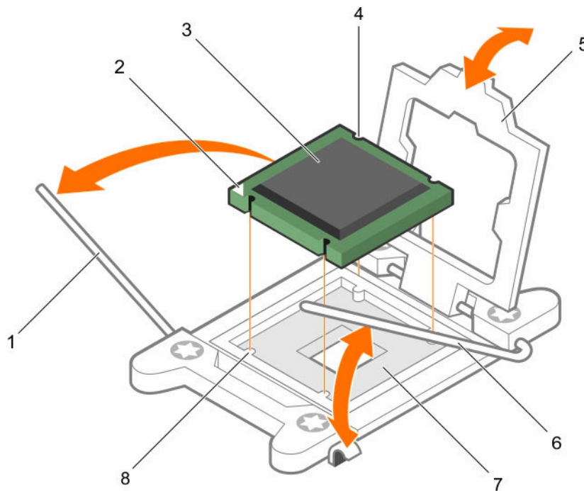
Abbildung 25. Entfernen und Einsetzen eines Prozessors
