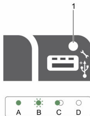
Abbildung 5. iDRAC Direct-LED-Anzeige
