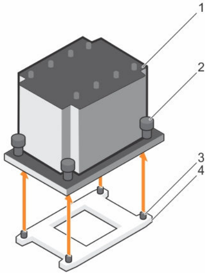
Abbildung 21. Entfernen und Einsetzen eines Prozessors
