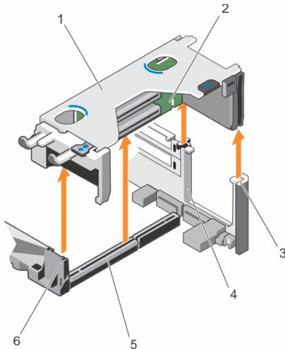
Abbildung 33. Entfernen und Einsetzen des Erweiterungskarten-Risers 1
