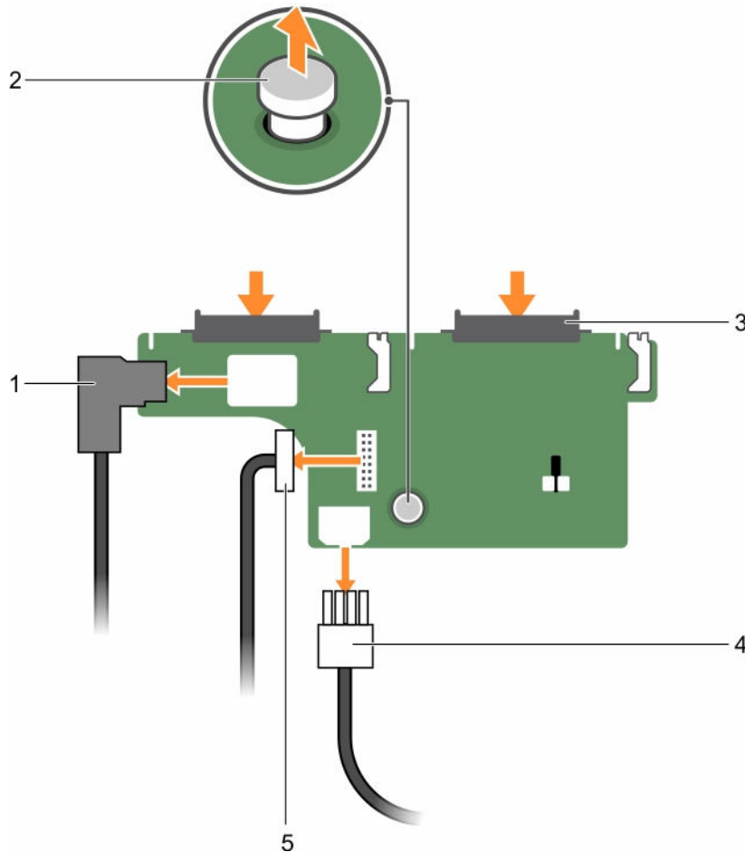
Abbildung 57. Entfernen und Installieren der optionalen 2,5-Zoll (x2) Festplatten-Rückwandplatine
