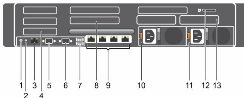
Abbildung 6. Funktionen und Anzeigen auf der Rückseite
