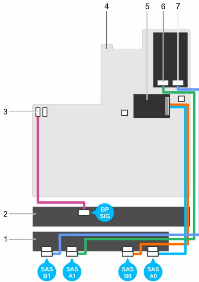
Abbildung 55. Verkabelungsschema – 2,5-Zoll(x24)-SAS/SATA-Rückwandplatine – (Option 2)
