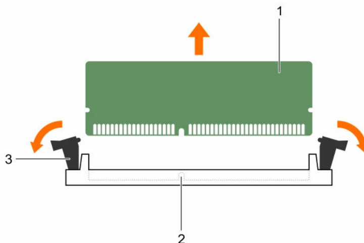
Abbildung 18. Entfernen und Installieren eines Speichermoduls
