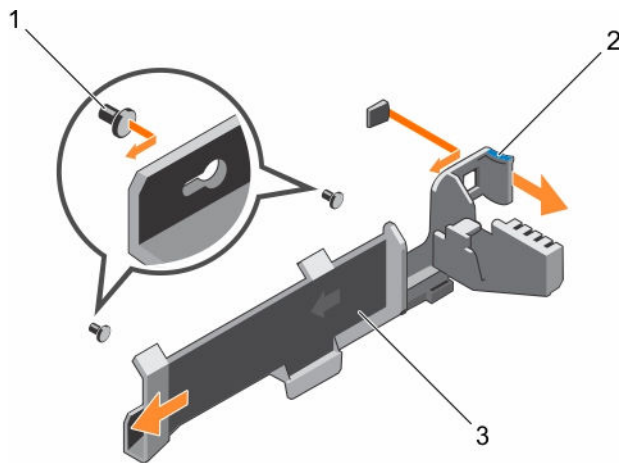
Abbildung 29. Entfernen und Einsetzen der Kabelhalteklammer
