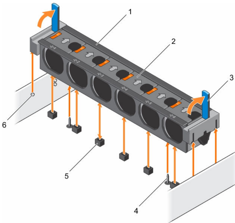
Abbildung 15. Entfernen und Installieren der Lüfterbaugruppe
