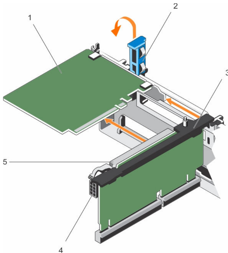
Abbildung 31. Entfernen und Einsetzen einer Erweiterungskarte aus dem Erweiterungskarten-Riser 2 oder 3
