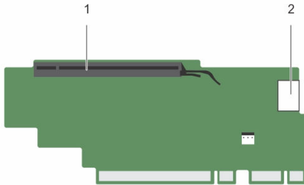
Abbildung 39. Identifizieren der Anschlüsse am Erweiterungskarten-Riser 3 (Alternativ)
