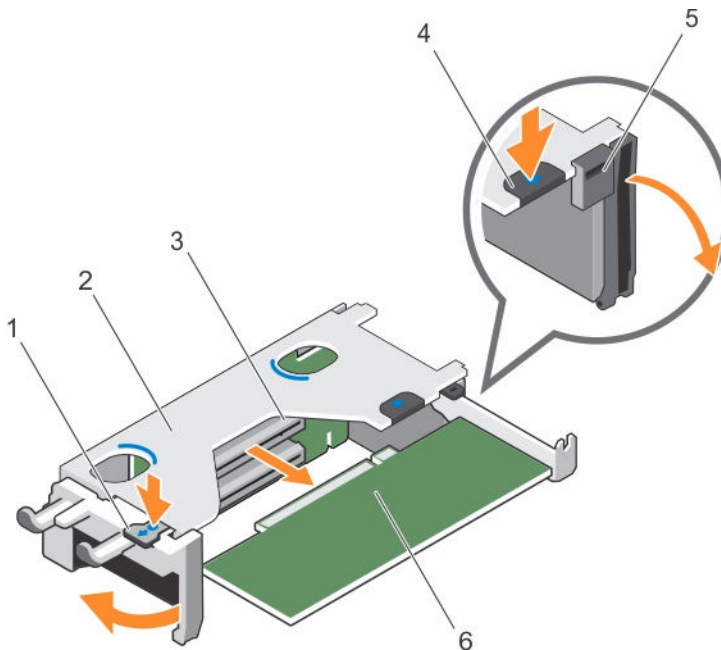
Abbildung 32. Entfernen und Einsetzen einer Erweiterungskarte in den Erweiterungskarten-Riser 1
