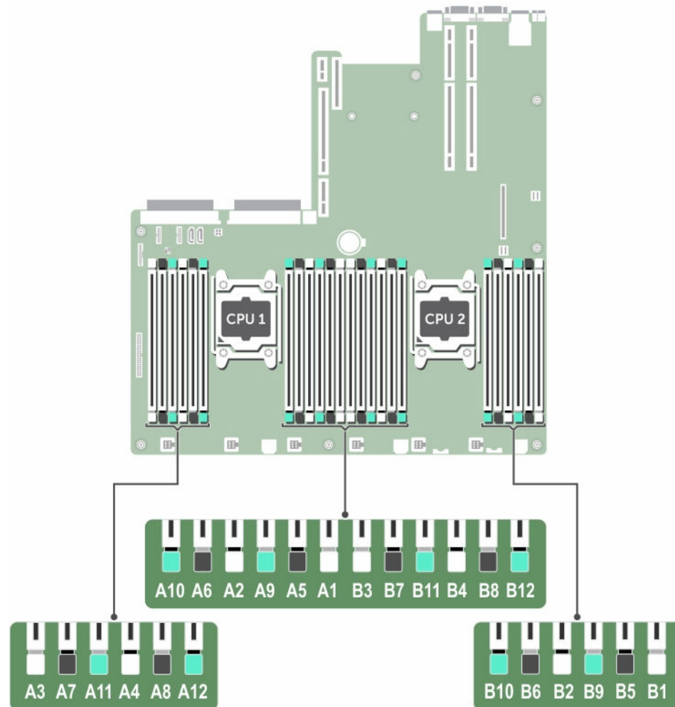
Abbildung 16. Positionen der Speichersocket
