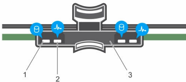
Abbildung 4. HDD-Anzeigen an der Rückwandplatine des Festplattenfachs
