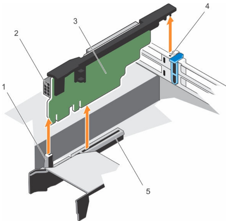
Abbildung 37. Entfernen und Einsetzen des Erweiterungskarten-Risers 3
