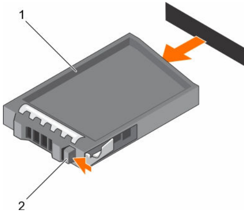
Abbildung 49. Entfernen und Einsetzen eines 2,5-Zoll-Festplattenplatzhalters
