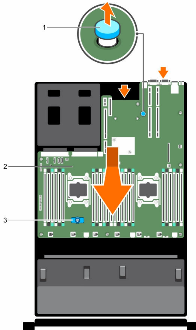
Abbildung 47. Entfernen und Einsetzen der Systemplatine
