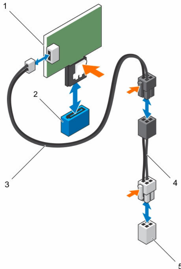
Abbildung 20. Entfernen und Installieren von SATADOM
