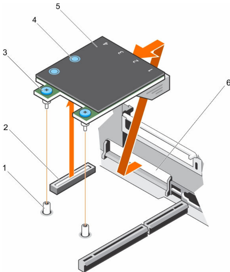
Abbildung 41. Entfernen und Einsetzen der Netzwerktochterkarte (NDC)
