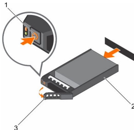
Abbildung 52. Entfernen und Installieren eines hot-swap-fähigen Laufwerks
