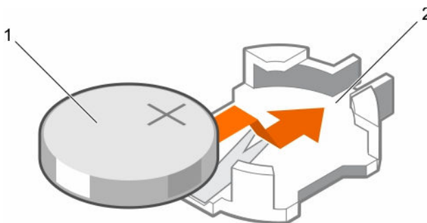
Abbildung 43. Installieren der Systembatterie
