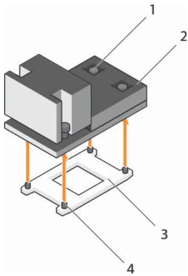
Abbildung 22. Entfernen und Einsetzen eines Prozessorkühlkörpers
